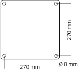
piani clienti, schema di foratura G02
